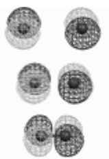
反結合性 \pi 軌道
