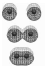
結合性 \pi 軌道
