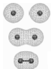
結合性 \sigma 軌道
