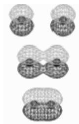
結合性 \pi 軌道
